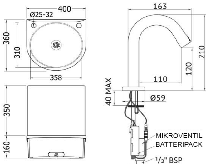
LEVERERAS MED TERMOSTATISK BLANDNINGS- VENTIL
